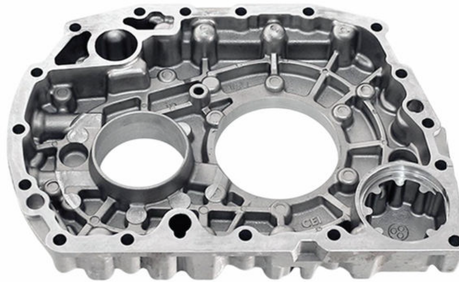
47 Housing ฝาหน้า, แผ่นเพสชนมป้รุ่น 330-360
